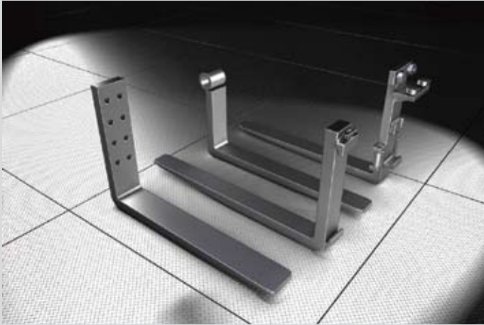
Forche standard e speciali di qualità con diversi agganci , ampia gamma di lunghezze e portate ma anche a vostro disegno .
