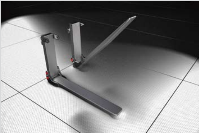
Forche pieghevoli di qualità per carrelli elevatori , macchine edili e agricole per ridurre gli ingombri e per macchine da cantiere che circolino anche su strada .
